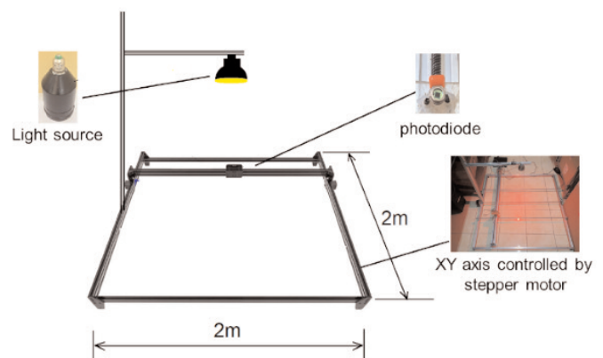
Hình 2. Hệ đo phân bố cường độ bức xạ của nguồn sáng LED
