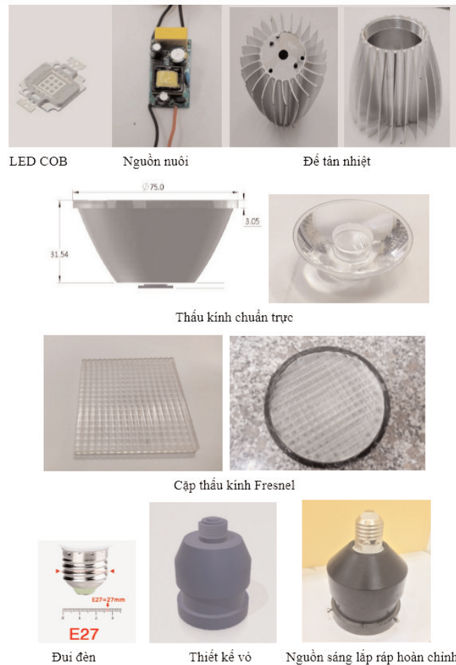
Hình 1. Các linh kiện trong nguồn sáng và nguồn đèn sau khi chế tạo hoàn chỉnh.
